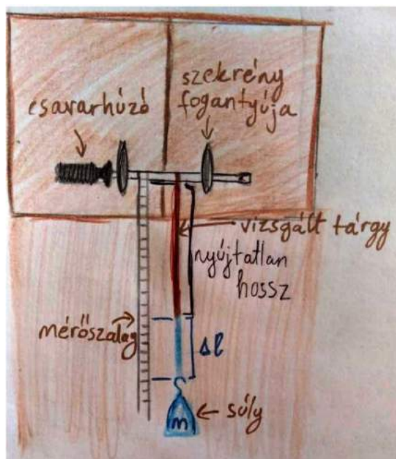
A 'kísérleti berendezés' vázlatos ábrája
